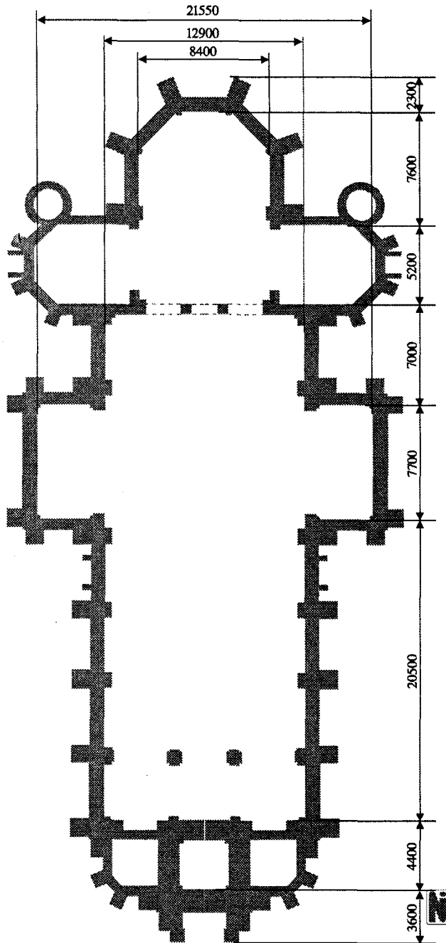
Az 1887 november 13-án felszentelt pécskai római katolikus templom alaprajza
