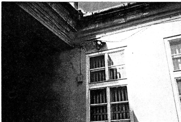
DEGRADARI PERETE AX J/12-13 > SONDAJ Nr. 2
