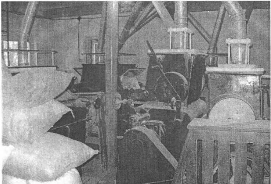
Az Oláh-farm: malom
