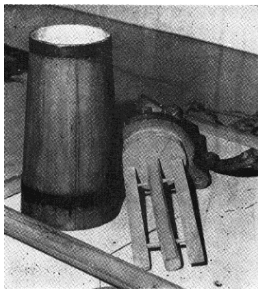
16—17. Fogaskerékáttétellel működő vajküpülő. BM
