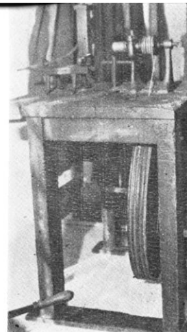
23. Kefefák faragására használt eszterga. BM
